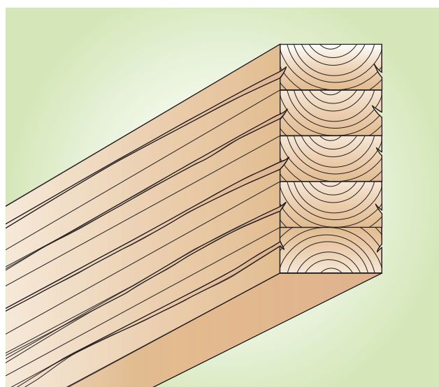
Richtige Balkenlage bei BS-Holz: rechte Seiten nach oben. Radiale Trockenrisse sollen nach unten verlaufen, damit sich keine Wassertaschen bilden.
