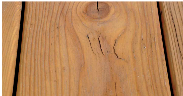
Schilfer/Ablösung der Jahrringe bei Nadelhölzern; darüber trocknungsbedingter Riss im gesunden Ast
