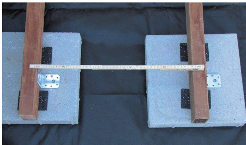
Ausrichten der Unterkonstruktion auf Platten
